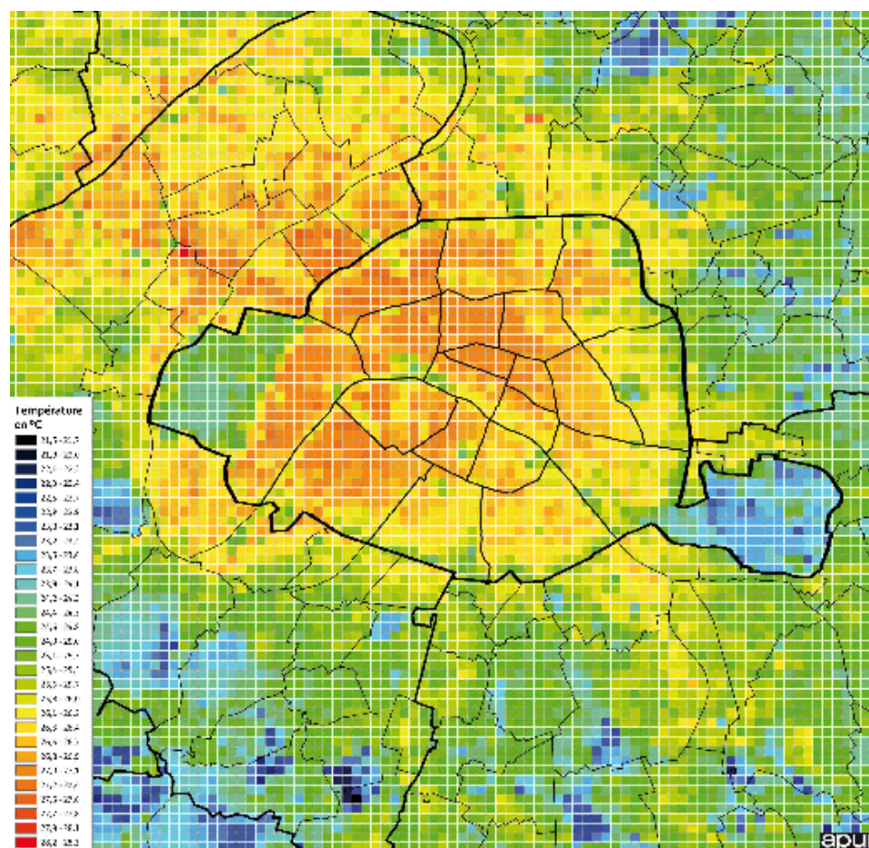
Figure 40. Les îlots de chaleur et les îlots de fraîcheur
